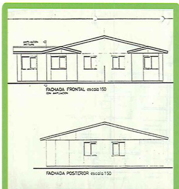
Plano con las fachadas frontal y posterior de las viviendas en Escritores de Chile.
